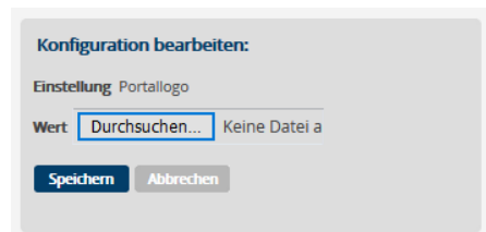
Bild 35: Portallogo hochladen
