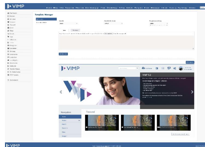
Bild 36: VIMP Template-Manager
