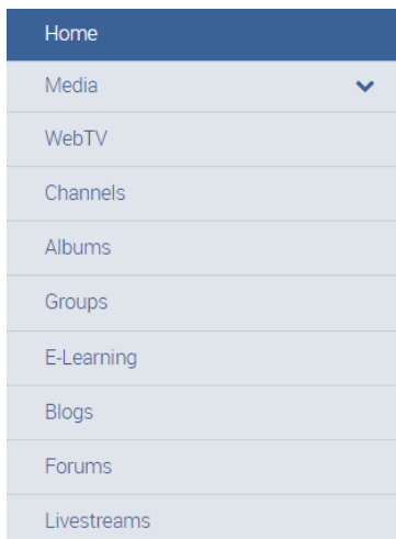
Bild 5: Navigations-Übersicht
