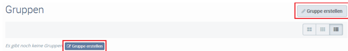
Bild 42: Gruppe erstellen
