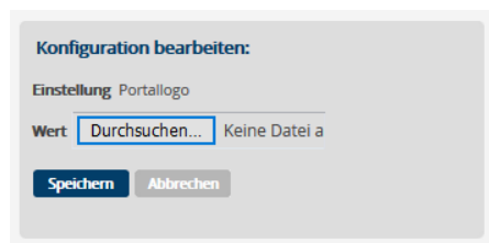
Bild 35: Portallogo hochladen
