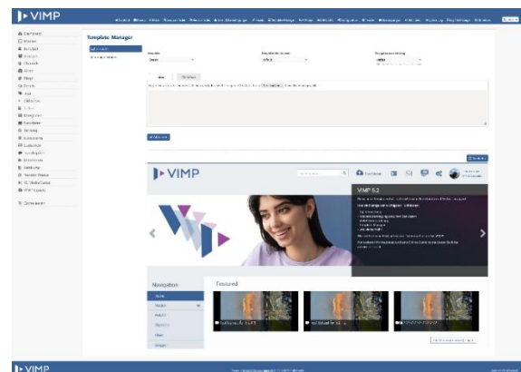
Bild 36: VIMP Template-Manager
