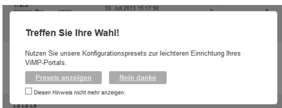
Bild 3: Preset-Hinweis
